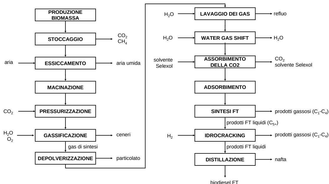
Figura 1: Schema a blocchi del processo di sintesi FT
