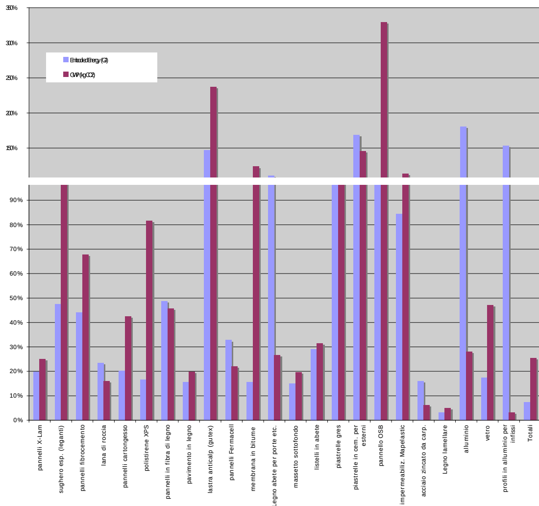
Figura 2: Massima variazione ((\max - \min) / \text{med}) degli impatti per i vari materiali utilizzati nel progetto, secondo i tre database "allineati": IBO, ECOINVENT, ITACA
