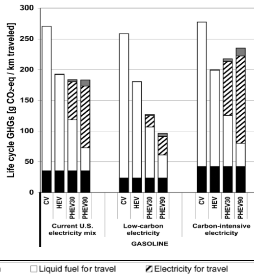
Figura 1: Risultati del confronto in termini di emissioni CO 2 lungo il ciclo di vita di 4 veicoli: uno tradizionale (CV) uno HEV e 2 PHEV. La costruzione del veicolo è identica nei 4 casi (fonte: Samaras, Meisterling 2008). I PHEV sono seguiti dai km di autonomia in modalità solo elettrica
